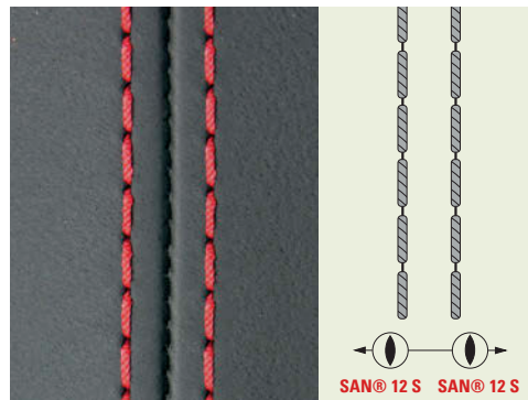
Pointe à tranchant S SAN® 12
